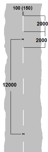
4 metre Module RRM 003B
