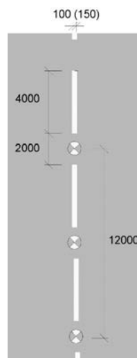
6 metre Module RRM 002C
