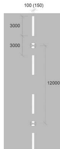
6 metre Module RRM 002B
