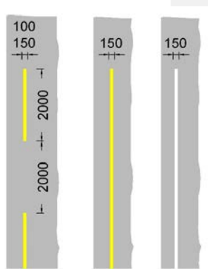
RRM 025 RRM 026 RRM 027
