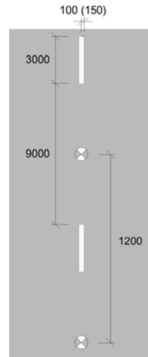
12 metre Module RRM 002A
