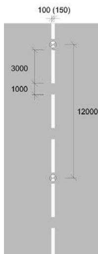
4 metre Module RRM 002D
